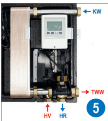
5 Installieren Sie die Heizungsanschlüsse und die Trinkwasseranschlüsse und spülen Sie die Station.
