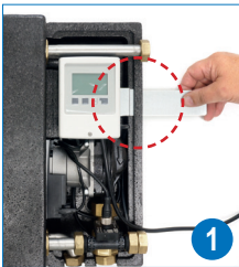
1 Befestigungsschiene von RECHTS her montieren.
